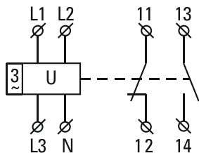
Рис. 4. Электрическая схема
